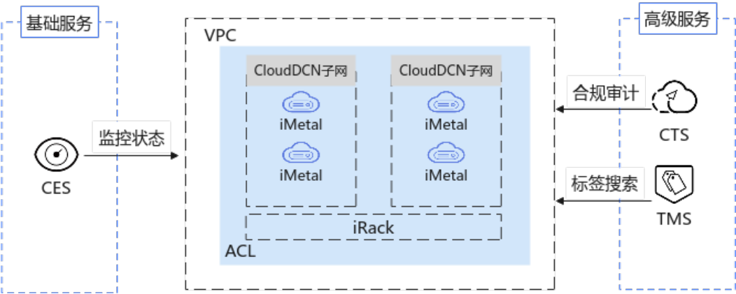
图 7-1 CloudDC 服务与其他服务的关系
